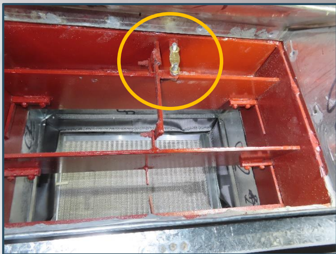
保險連桿
